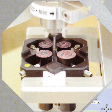
マルチバイス (丸) で 代表印を4本連続彫刻 ※オプション
